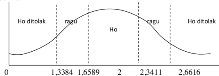
Gambar 4 Grafik Durbin-Watson
